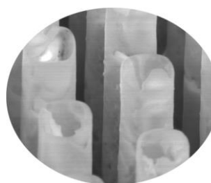
Nanorurki ferroelektryczne
